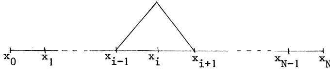
Figuur 2.3 Grafiek van \phi_i(x) .
