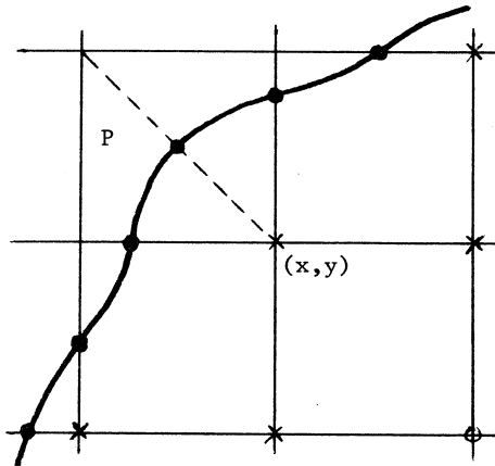
Figuur 1.6 Niet-inwendig randpunt (x,y)
