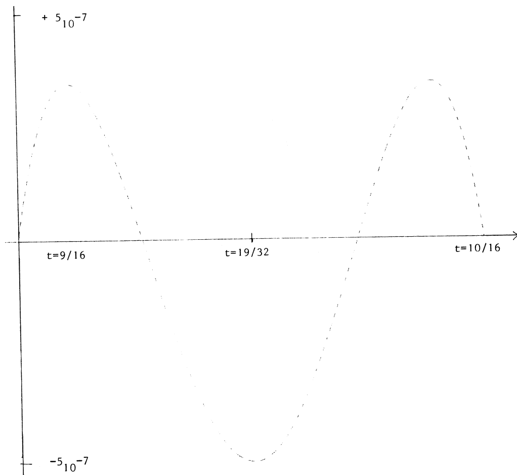
Figuur 5.3 grafiek I.
