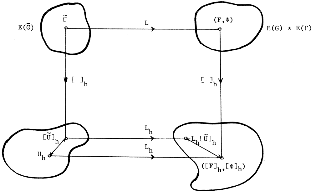
Figuur 1.4 Afbrekfout en discretiseringsfout
