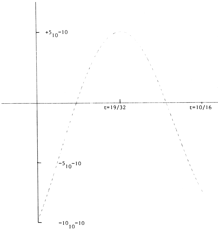
Figuur 5.5 grafiek III.
