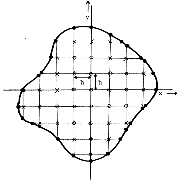
Figuur 1.5 Vierkant rooster met maaswijdte h
