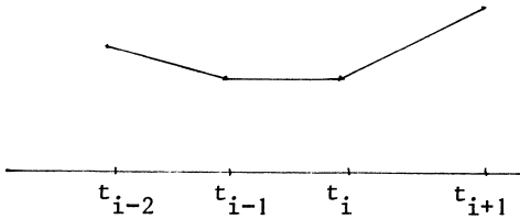
Figuur 5.1 Element uit E(\delta_N; 1)
