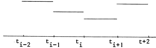
Figuur 5.2 Element uit F(\delta_N; 0)
