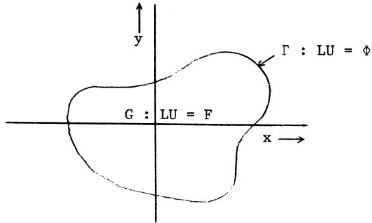
Figuur 1.1 Randwaardeprobleem
