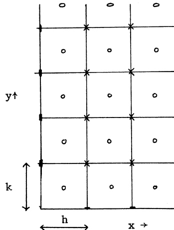
Figuur 1.8 Stromingspunten (x, -, l) en verhogingspunten in rechthoekig Noordzeemodel.
