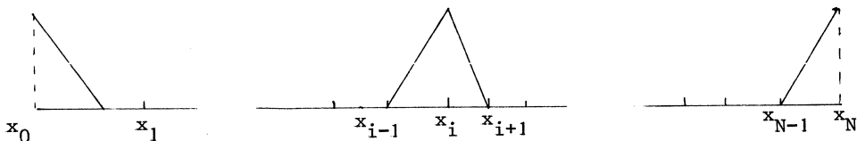
Figuur 3.2 Dakfuncties \phi_i(x)
