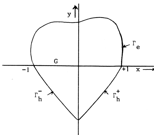
Figuur 1.2 Tricomi-probleem
