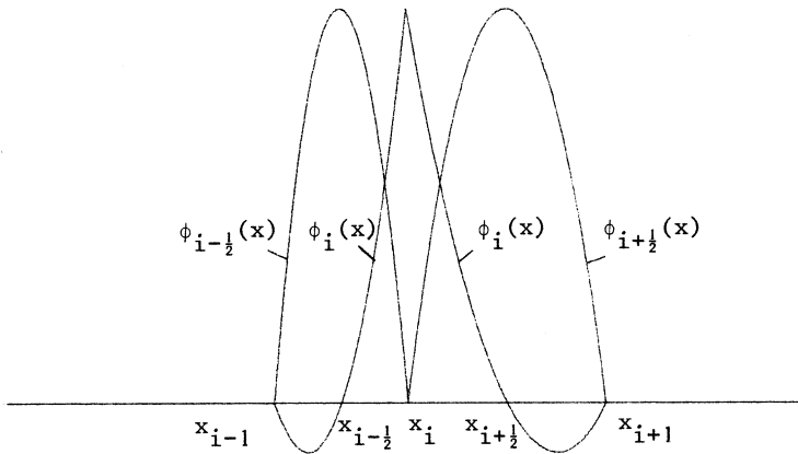
Figuur 3.4 Grafiek van \phi_{i-\frac{1}{2}}(x) , \phi_i(x) en \phi_{i+\frac{1}{2}}(x)
